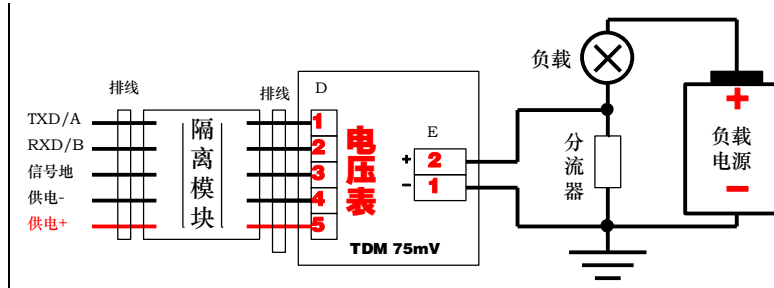
图 412 不要忽略隔离模块的作用
