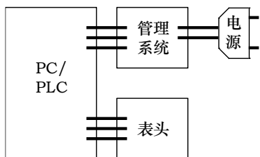
图 408 非隔离并联供电和通信
