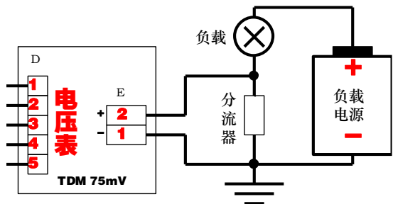
图 410 低端接入分流器测量电流
