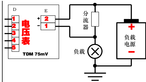
图 411 高端接入分流器测量电流
